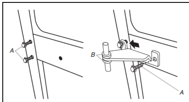
A. Vis de charnière à tête hexagonale de 5/16 po
